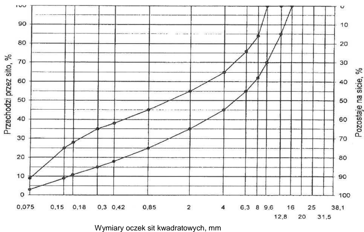
Rys. 10. Krzywe graniczne uziarnienia mieszanki mineralnej BA od 0 do 12,8 mm do warstwy wiążącej, wyrównawczej i wzmacniającej nawierzchni drogi o obciążeniu ruchem KRI lub KR2
